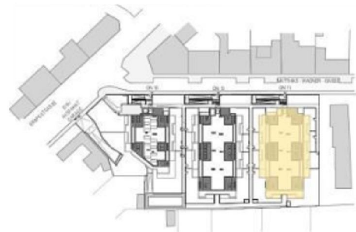
LAGEPLAN
