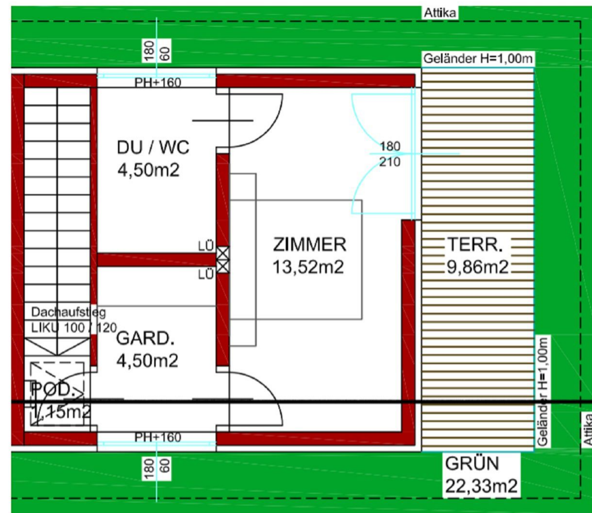
DACHGESCHOSS
