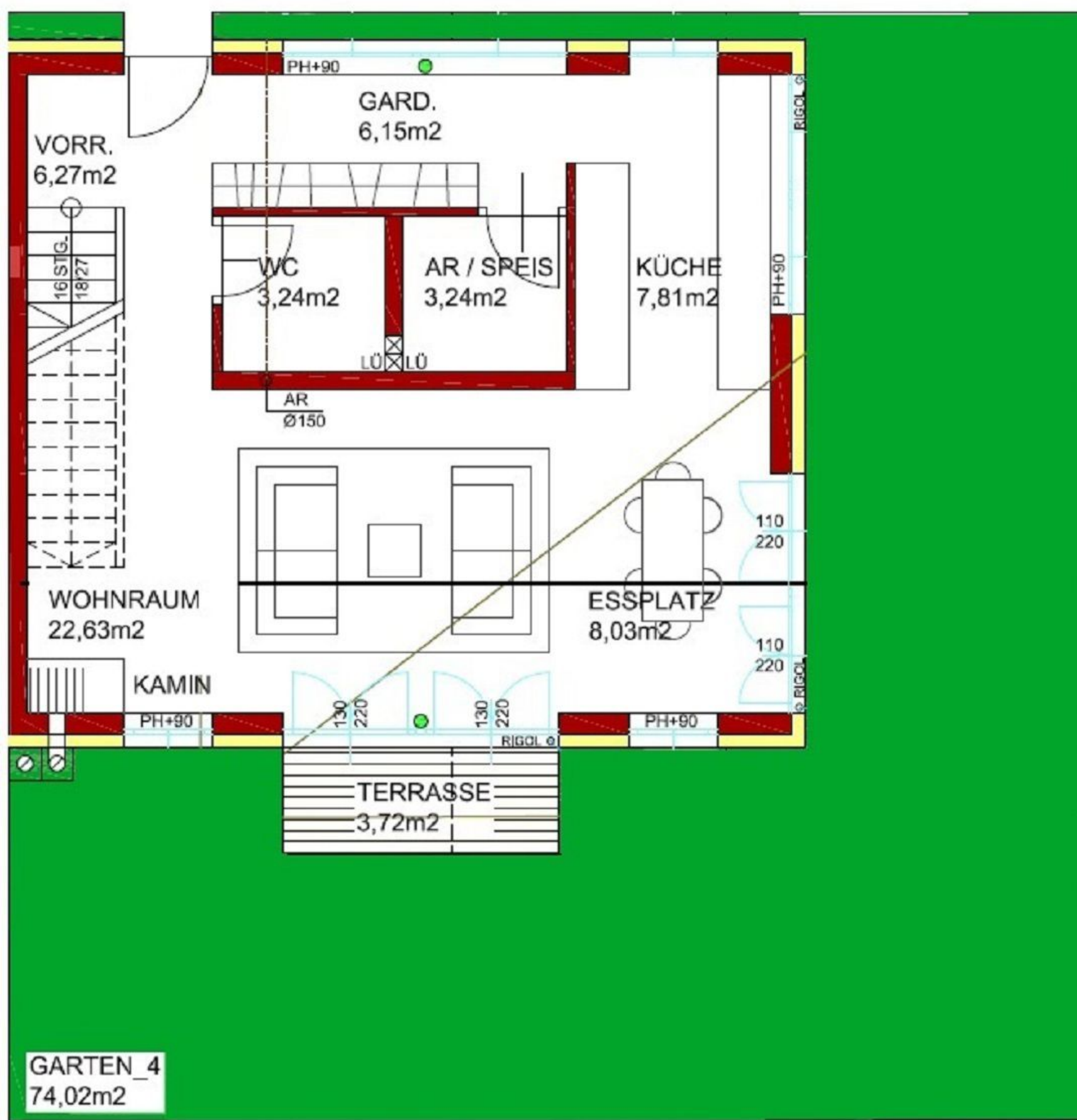
ERDGESCHOSS
