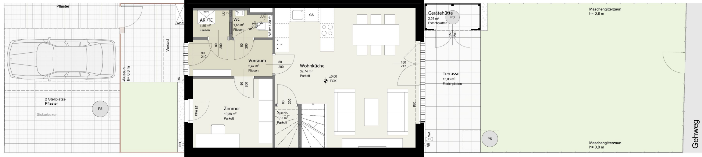
ERDGESCHOSS
