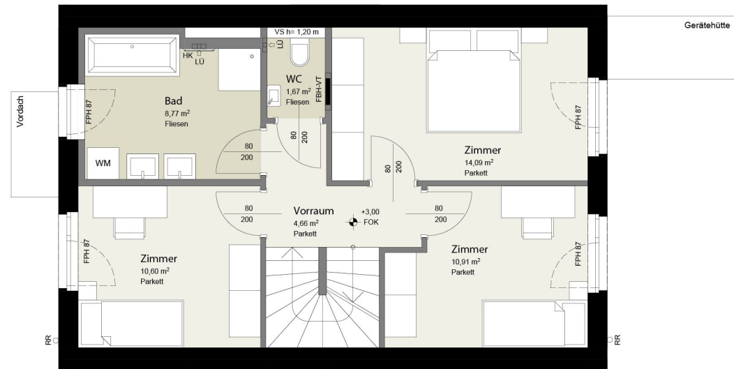
1.OBERGESCHOSS
