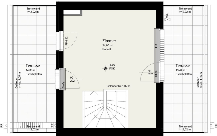
DACHGESCHOSS
