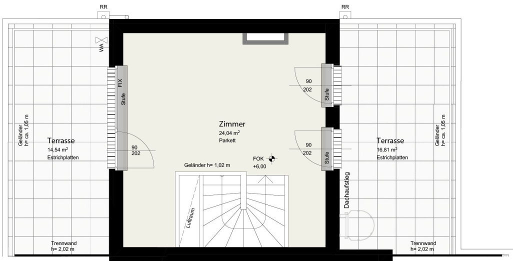
DACHGESCHOSS
