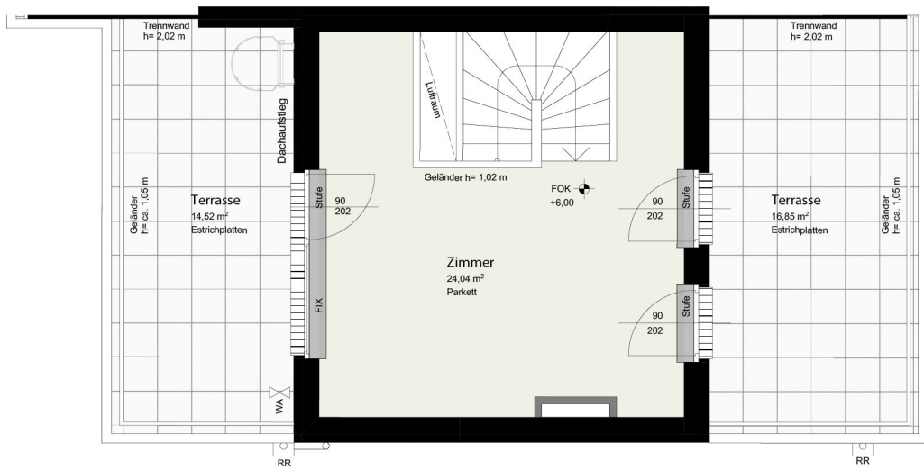
DACHGESCHOSS
