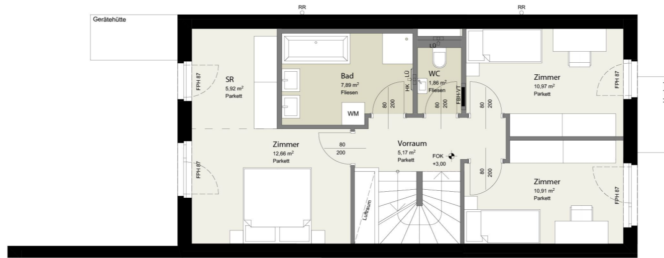
1.OBERGESCHOSS
