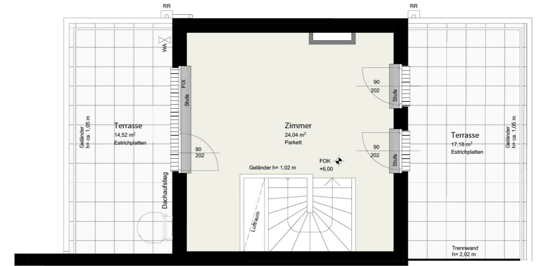
DACHGESCHOSS
