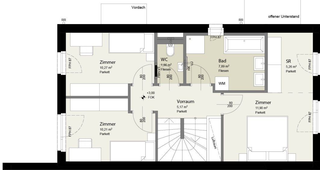
1.OBERGESCHOSS
